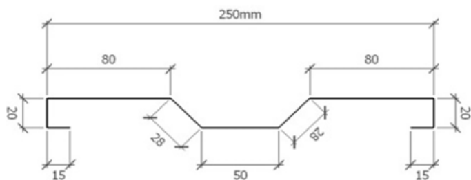
Элемент ограждения
